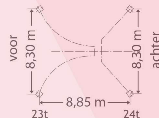
stempelbreedte
